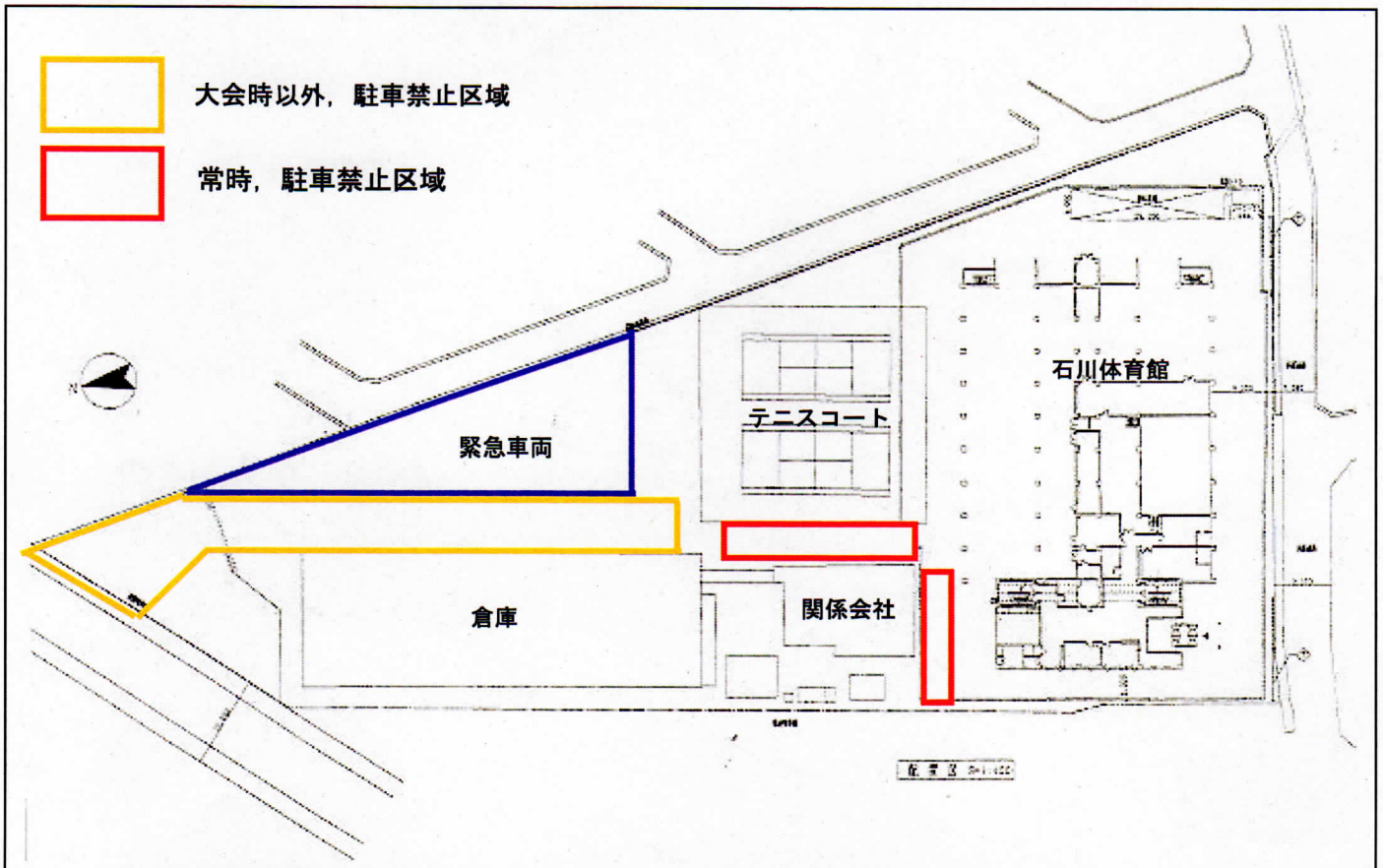
平面図
